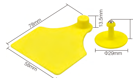
LD-7858A 9g/set
